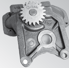
اویل پمپ 399
